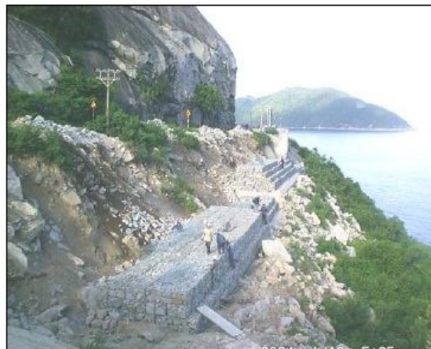
Tường chắn rọ đá trên đèo Cả -Đoạn cua Đá Đen – Dự án Cải tạo Quốc lộ 1A ADB3
